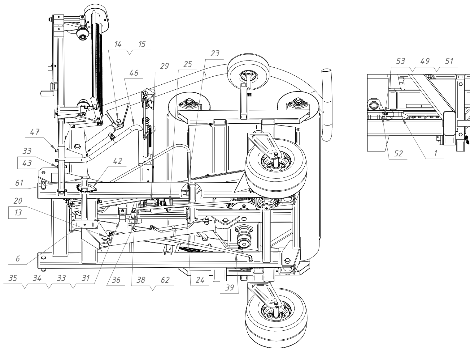
Tablica 2 5557-000-000.10 Owijarka kpl. /cz. 2/
