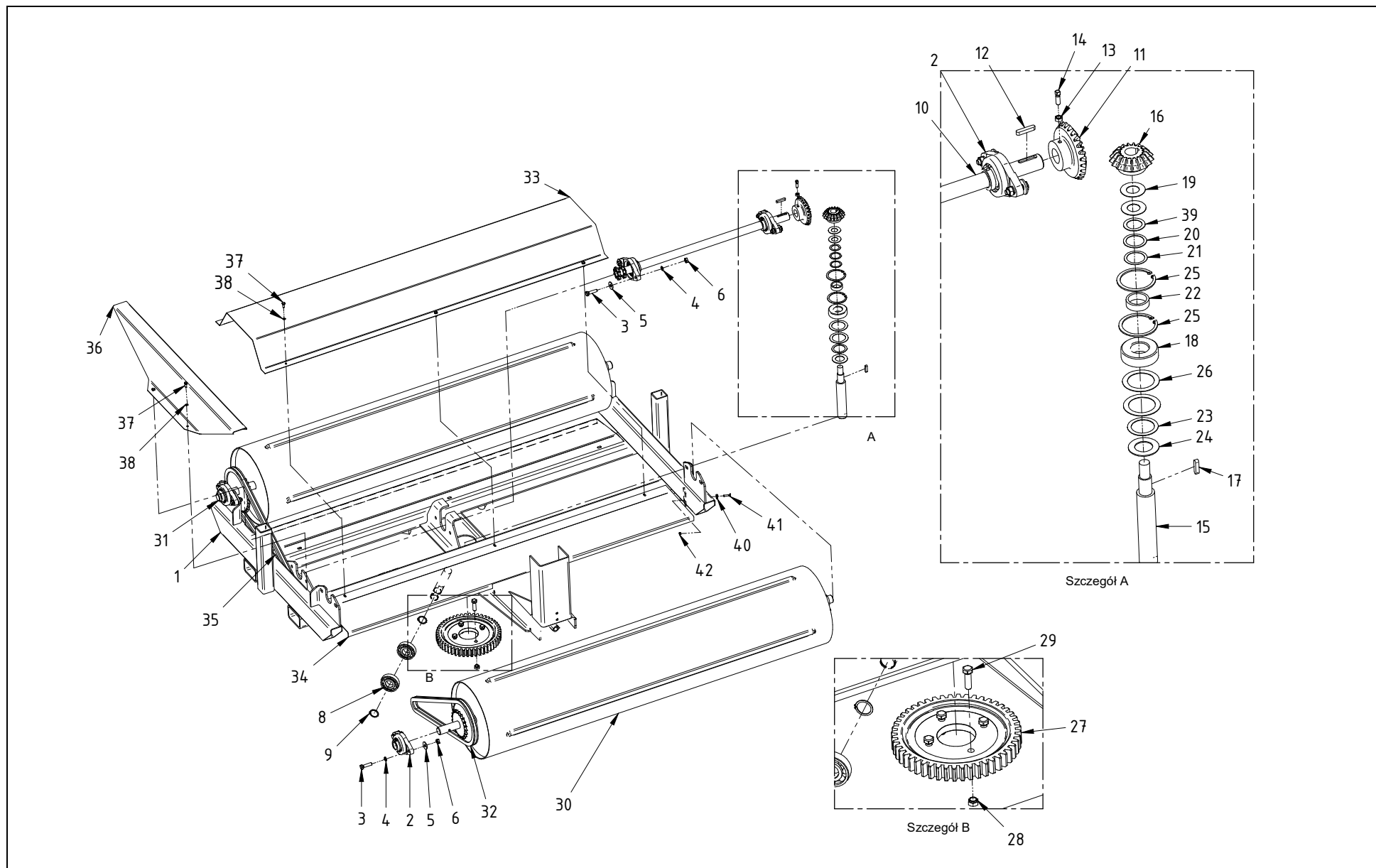
Tablica 3 5557-030-500.00 Rama obrotowa kpl.
