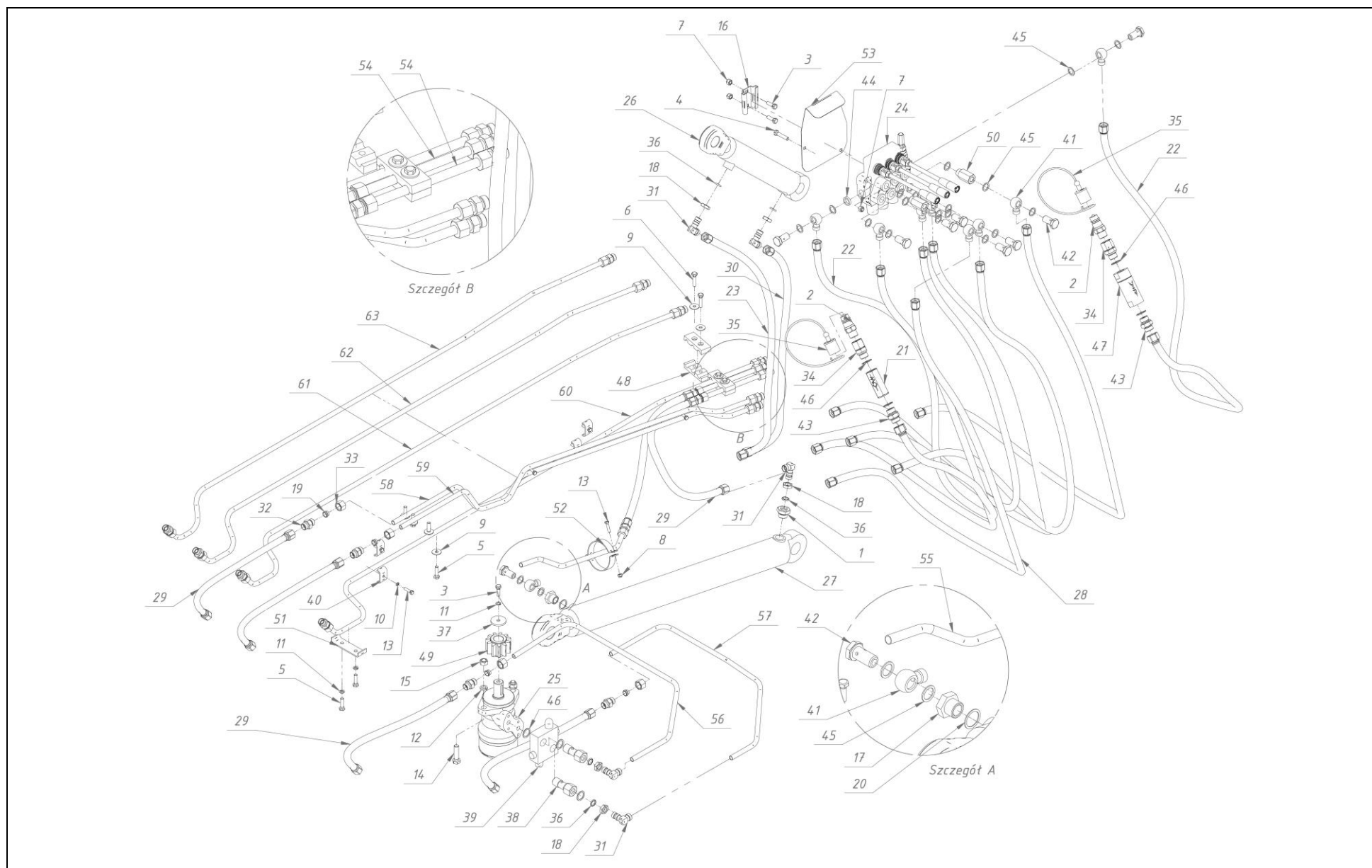
Tablica 5 5557-050-500.10 Instalacja hydrauliczna
