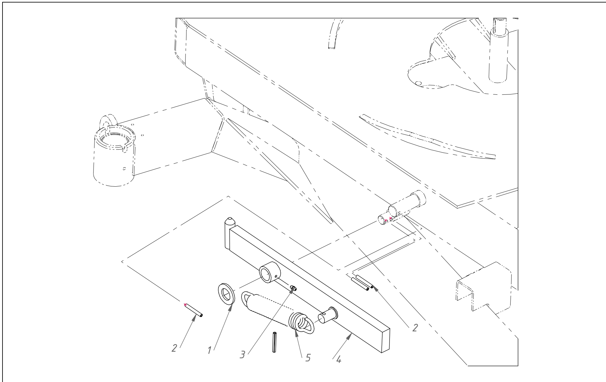
Tablica 4 5557-030-590.00 Blokada kpl.
