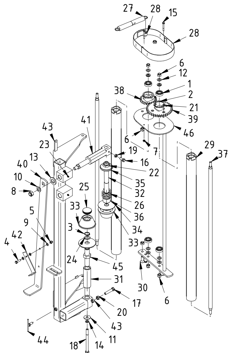
Tablica 8 5281-080-550.31 Podajnik folii 500-750
