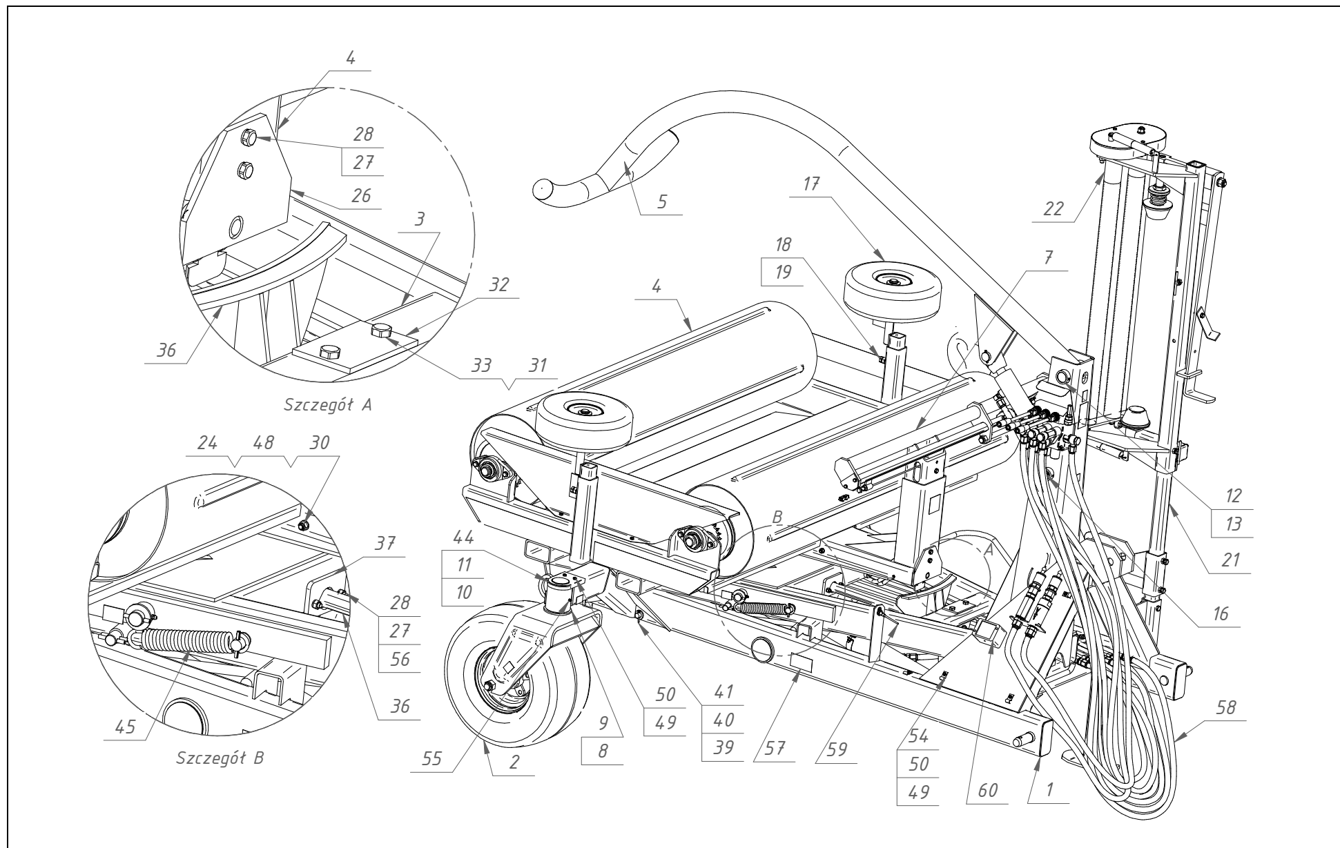
Tablica 1 5557-000-000.10 Owijarka kpl. /cz. 1/
