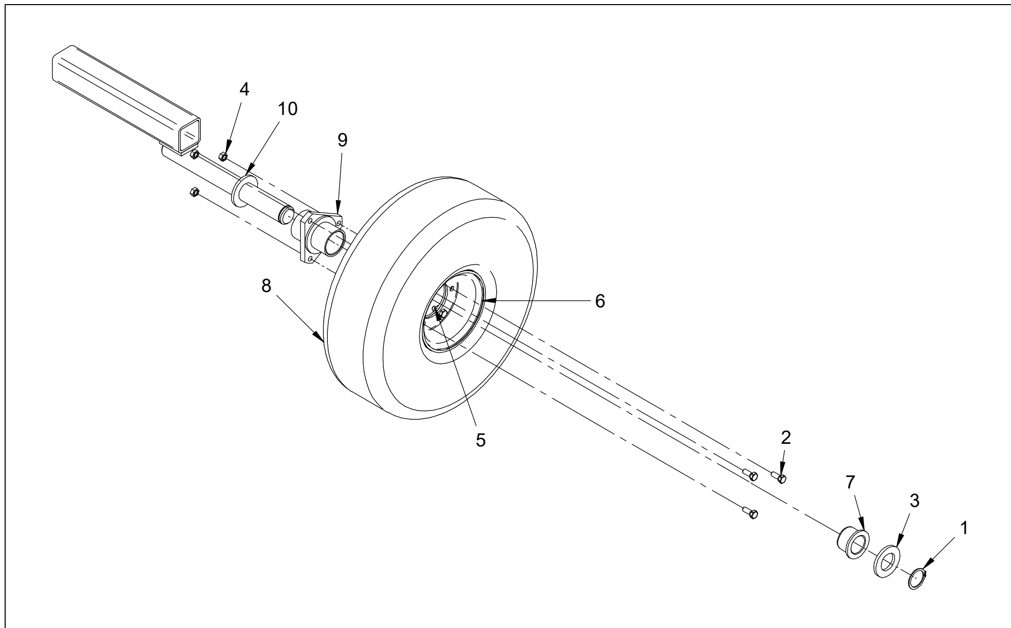
Tablica 9 1600-060-500.00 Kolo kpl.
