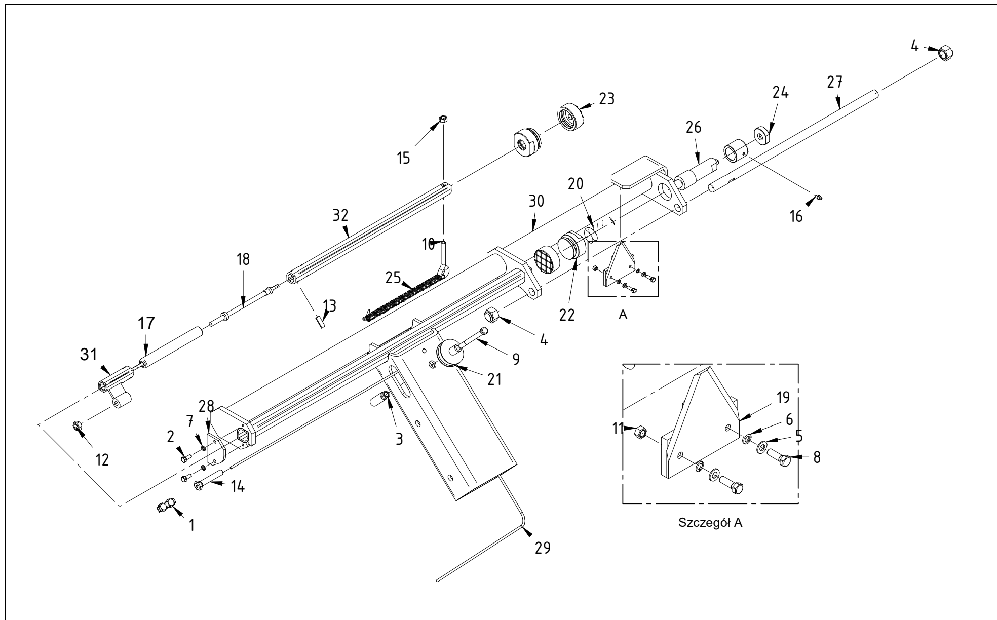
Tablica 7 5557-070-500.00 Chwytnik folii kpl.
