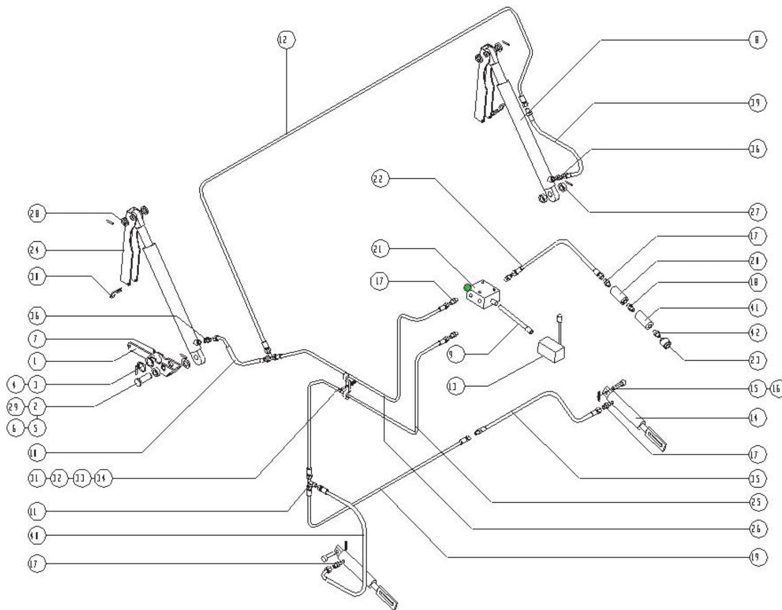
Гидравлическая система
