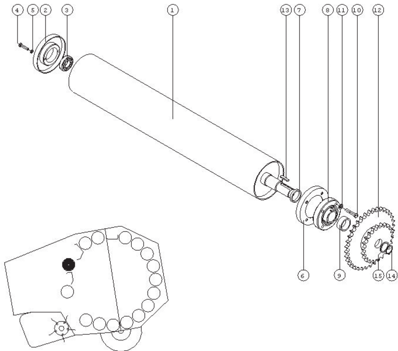
Прессующий вал в сборе IV
